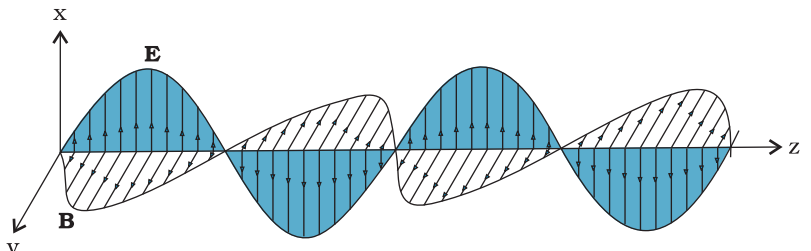
चित्र 8.3 एक रेखीय ध्रुवित वैद्युतचुंबकीय तरंग जो z -दिशा में गमन कर रही है और जिसका दोलनकारी विद्युत क्षेत्र E , x -दिशा के अनुदिश एवं दोलनकारी चुंबकीय क्षेत्र B , y -दिशा के अनुदिश है।
