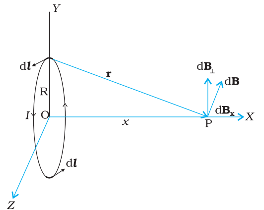
चित्र 4.9 त्रिज्या R विद्युत धारावाही वृत्ताकार पाश के अक्ष पर चुंबकीय क्षेत्र। इस चित्र में रेखा अवयव d\mathbf{l} के कारण चुंबकीय क्षेत्र d\mathbf{B} तथा अक्ष के लंबवत कार्यरत इसके अवयवों को दर्शाया गया है।
