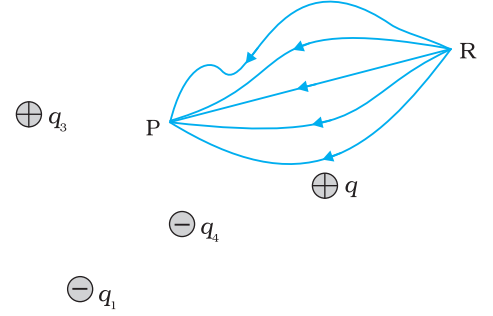
चित्र 2.2 किसी आवेश विन्यास के कारण स्थिरवैद्युत क्षेत्र द्वारा परीक्षण आवेश q पर किया गया कार्य पथ पर निर्भर नहीं करता, यह केवल अंतिम तथा आरंभिक स्थितियों पर निर्भर करता है।
