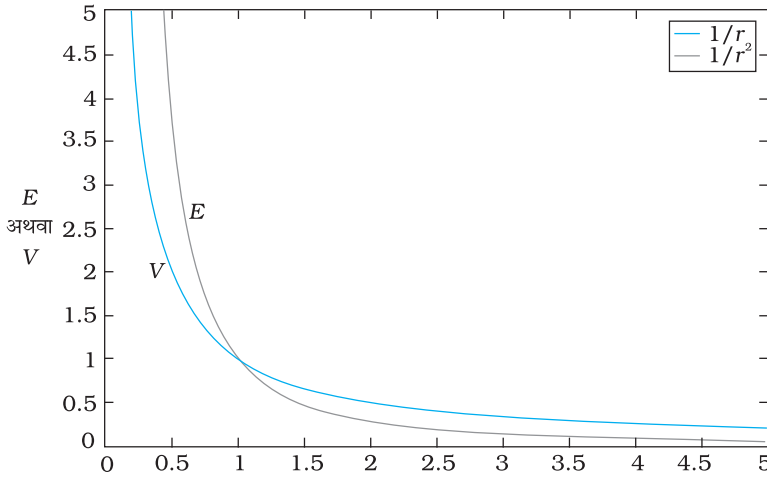
चित्र 2.4 किसी बिंदु आवेश Q के लिए दूरी r में परिवर्तन के साथ विभव में परिवर्तन ( Q/4\pi\epsilon_0 ) m^{-1} के मात्रकों में (नीला वक्र) तथा दूरी r में परिवर्तन के साथ विद्युत क्षेत्र में परिवर्तन ( Q/4\pi\epsilon_0 ) m^{-2} काला वक्र।
