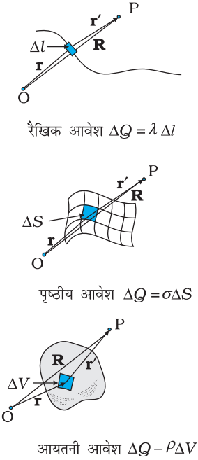
चित्र 1.21 रैखिक, पृष्ठीय, आयतनी घनत्वों की परिभाषा। प्रत्येक प्रकरण में चुने गए अवयव ( \Delta l, \Delta S, \Delta V ) स्थूलदर्शीय स्तर पर छोटे हैं परंतु इनमें सूक्ष्मदर्शीय स्तर के अवयवों की एक विशाल संख्या समाहित होती है।
