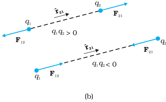
चित्र 1.3 (a) ज्यामिति तथा (b) आवेशों के बीच आरोपित बल।
